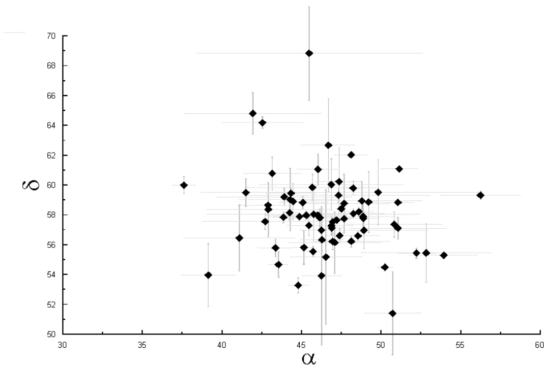
Indywidualne radianty dla perseidów bazowych
